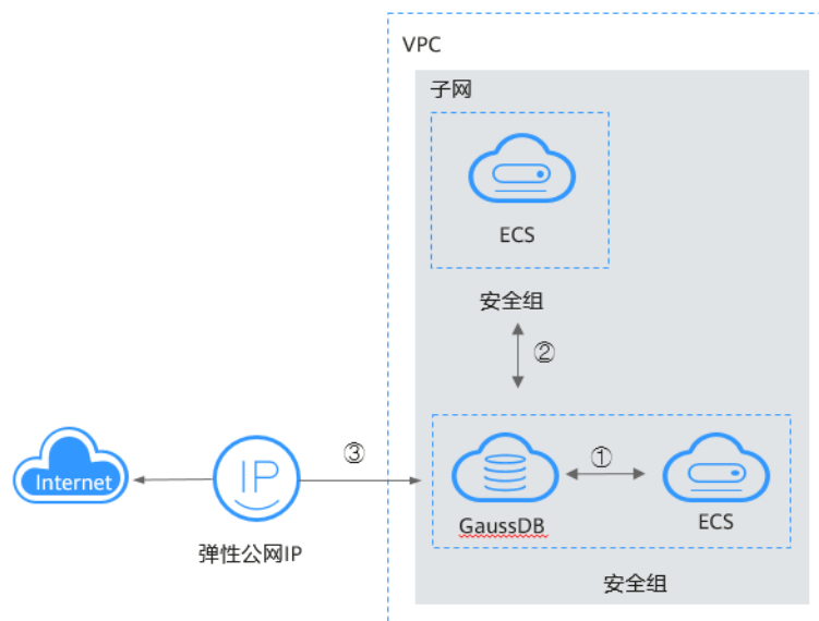
图 3-1 实例内网和弹性公网连接
