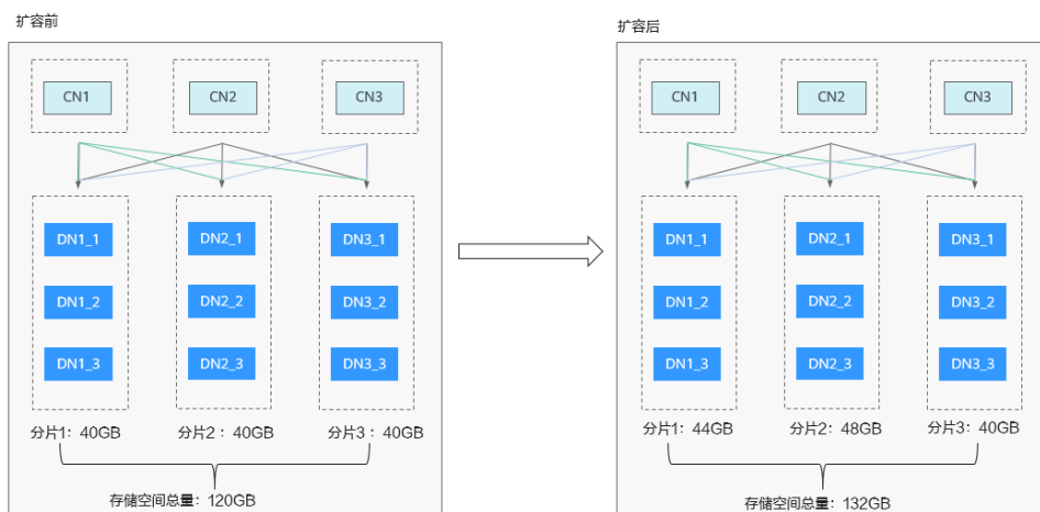
图 7-19 扩容示意图
