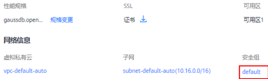
图 6-2 网络信息
