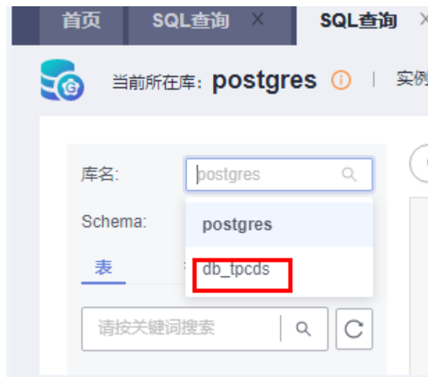
图 8-19 切换数据库
