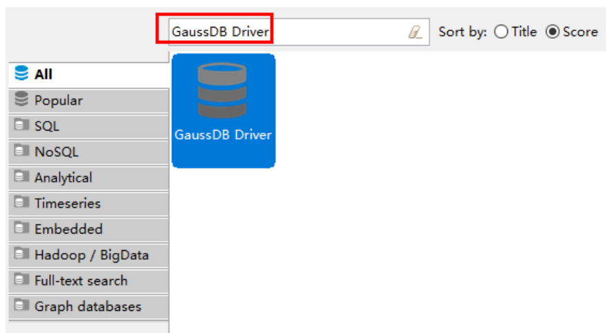
图 3-13 选择驱动
