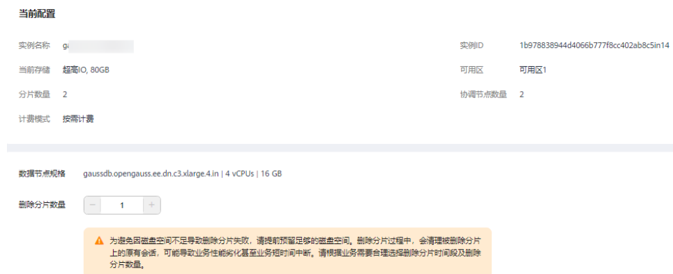
图 7-17 分片缩容
