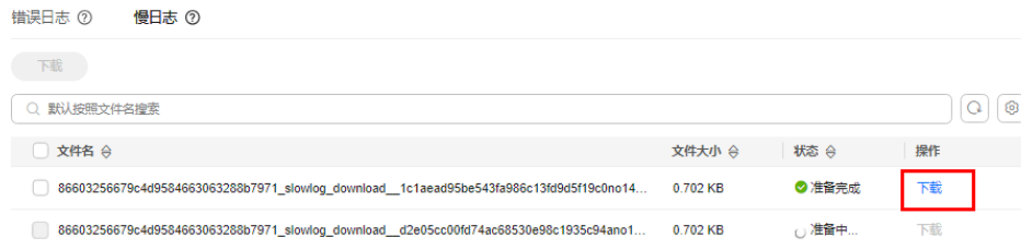
图 14-1 慢日志下载
