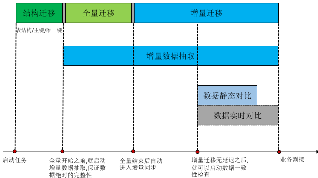
图 4-1 迁移原理图
