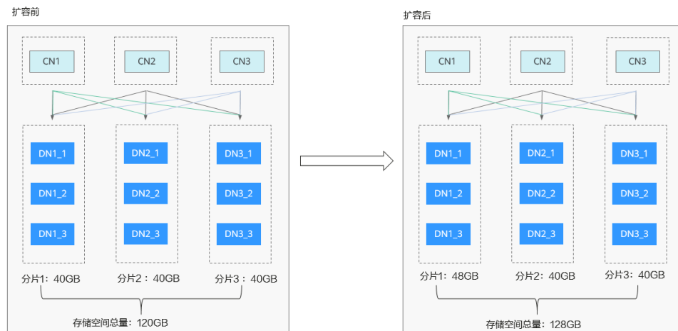
图 7-20 扩容示意图
