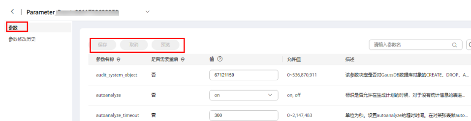
图 12-2 修改参数
